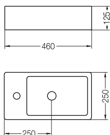
Lavatorio Tori Toilette 250 x 460 - 1 Agujero LK302 B
