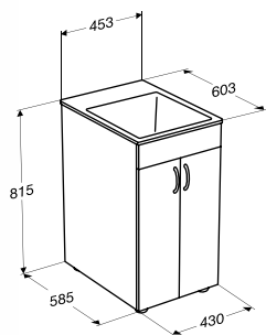
Conjunto pileta de lavadero rectangular y mueble laqueado blanco (armado) YL20A SB
