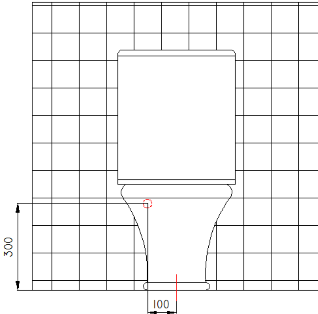
Esquema / de instalación de flexible recomendado
